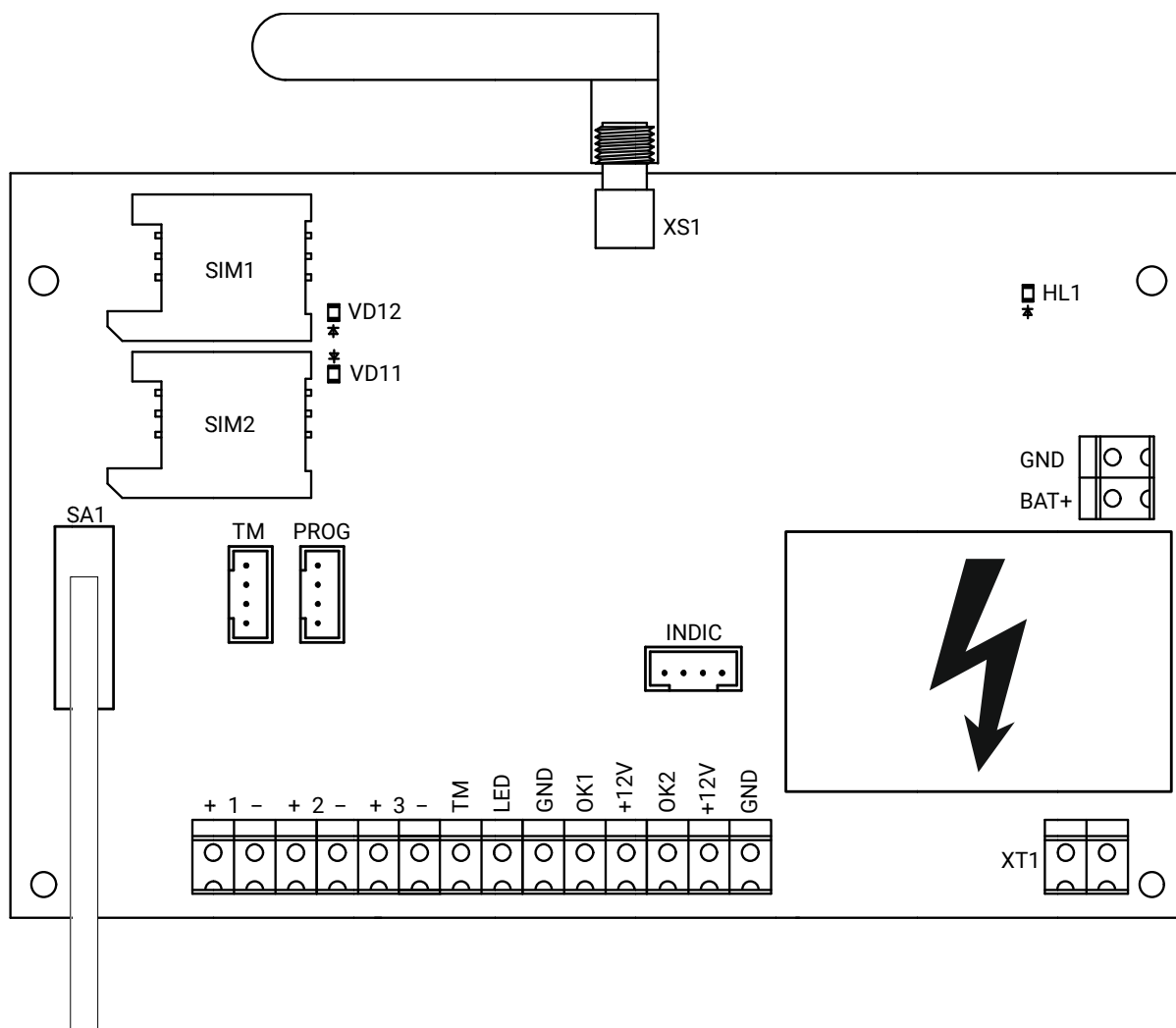
Рисунок 1. Плата прибора
