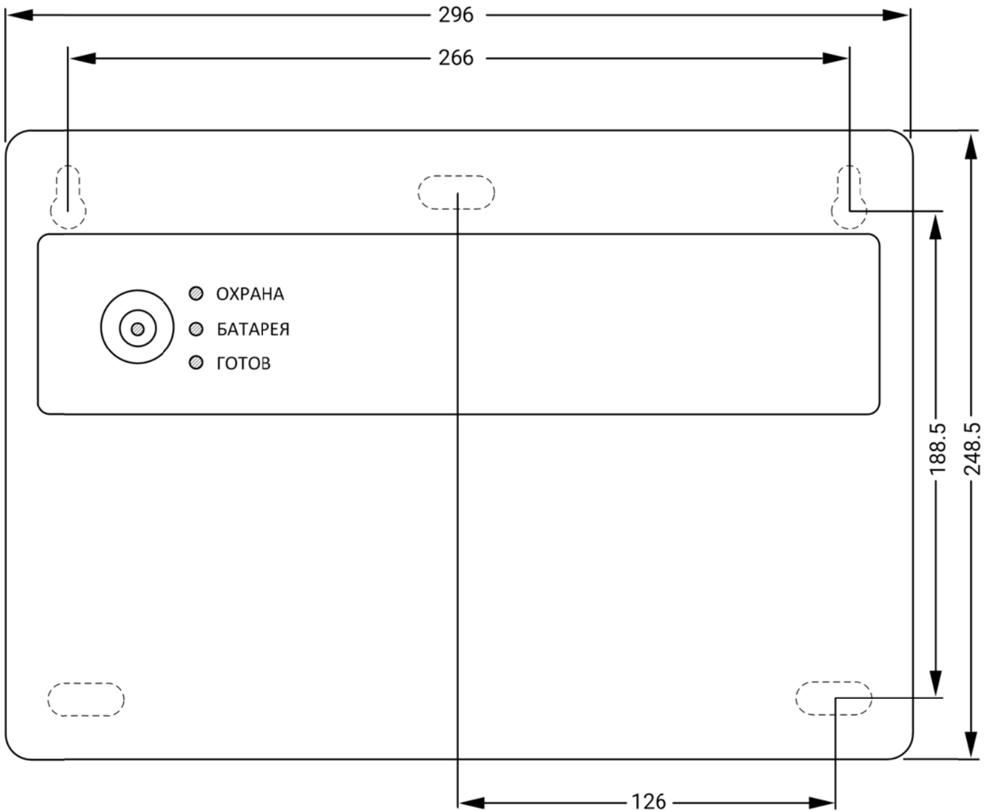
Рисунок 3. Корпус «Контакт 7 Ач» 3
