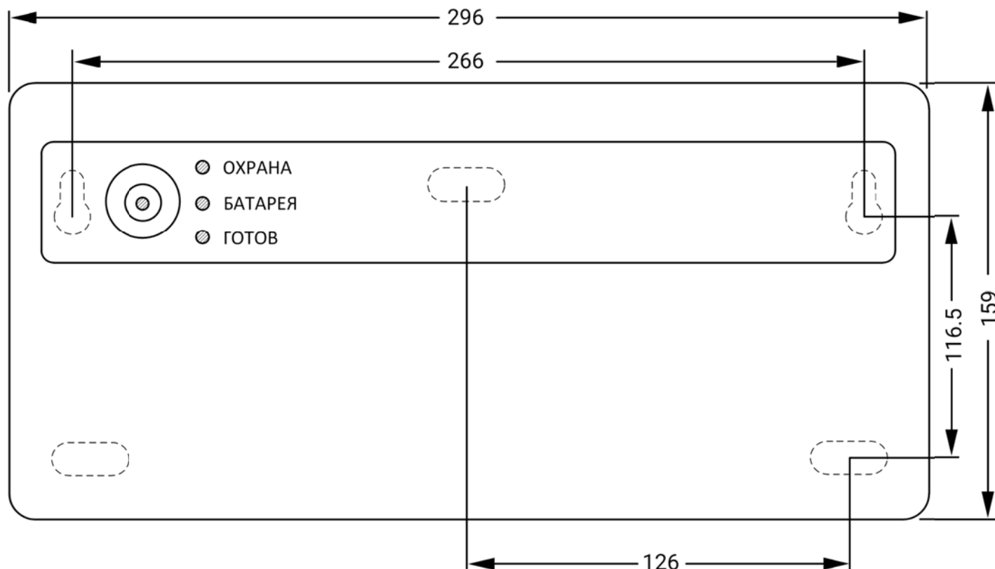
Рисунок 2. Корпус «Контакт 1.2 Ач»
